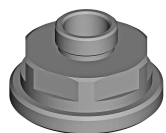
ZGHI027 Ecrou de fixation pour inverseur M37x1.5 pour art. 018-019 M37x1.5 Bevestigingsmoer voor omsteller voor art. 018-019
