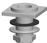
ZBAS085 Set de base complet (bague, embase et fixation) pour douchette pour art. 040-041 Complete basisset (ring, basis en bevestigingsset) voor handdouche voor art. 040-041
