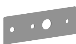
ZPIA056 Plaque murale 4 trous avec joints pour art. 001/ L.350 x h.120 mm 4-gatsmuurplaat met dichtingen voor art. 001/ L.350 x h.120 mm
